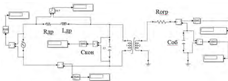
Рис.4. Схема моделирования в Matlab.
